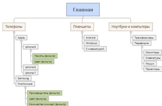
Рисунок 4-Структура сайта
